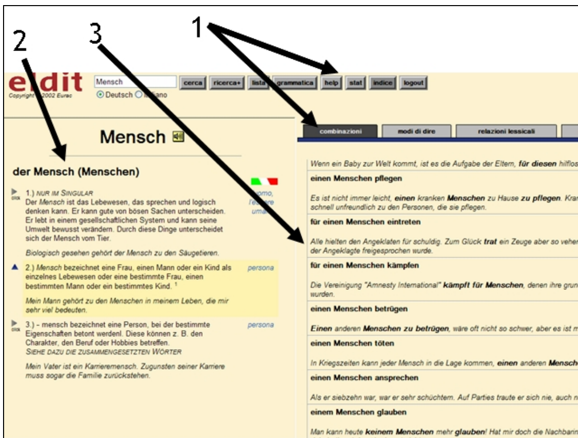
Abbildung 2: Benutzeroberfläche ELDIT
